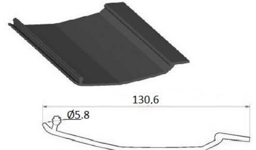
Çatı Lastiği Code DMR.11 Pvc Pelmet Code DMR.11
