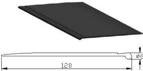
Çatı Lastiği Code DMR.10 Pvc Pelmet Code DMR.10
