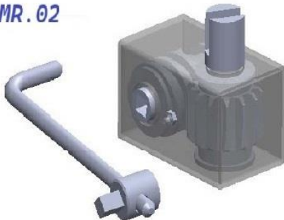
Branda Gerdirme Aparatı Ratchet
