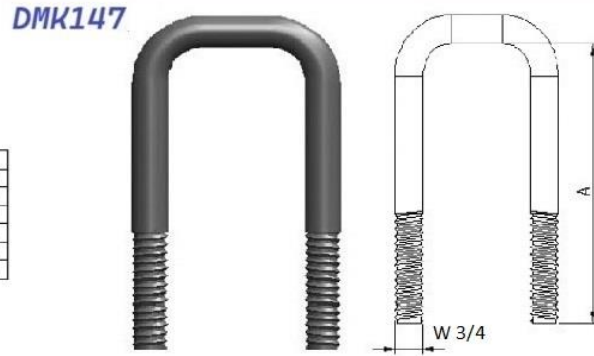
Trailer bağlantı Trailer connection
