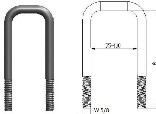
Kasa bağlantısı Van connection
