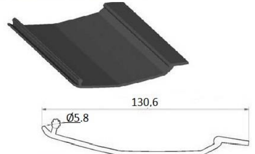
Çatı Lastiğ Code DMR.11 Pvc Pelmet Code DMR.11
