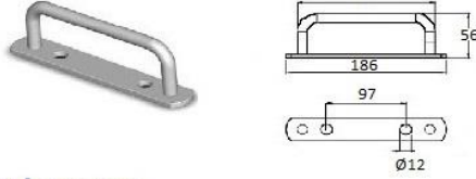
El tutamagı Hand Grip
