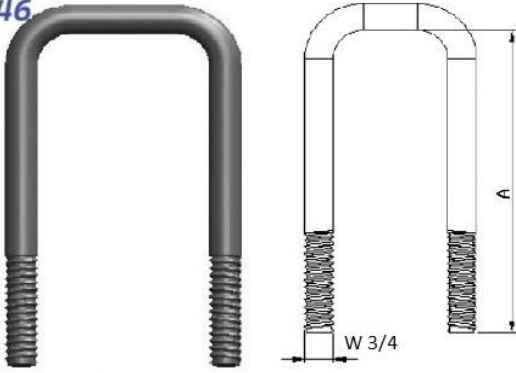
Damper bağlantı Dumper connection
