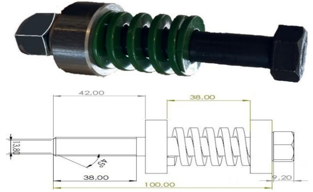
Şase bağlantı Vidası Chasses Connection Screw
