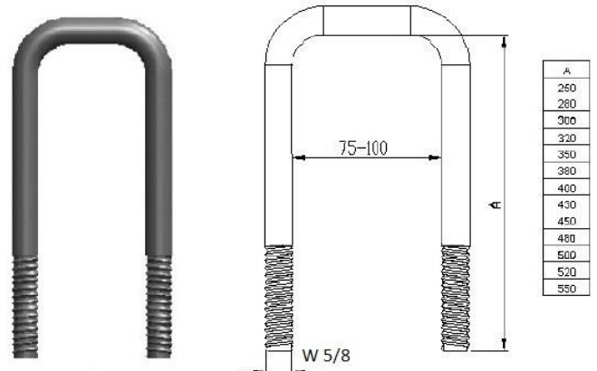
Kasa bağlantısı Van connection
