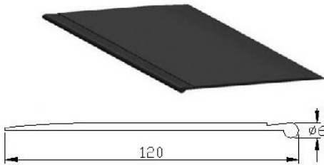
Çatı Lastiği Code DMR.10 Pvc Pelmet Code DMR.10
